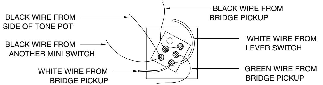
DETAIL " B " MINI SWITCH
